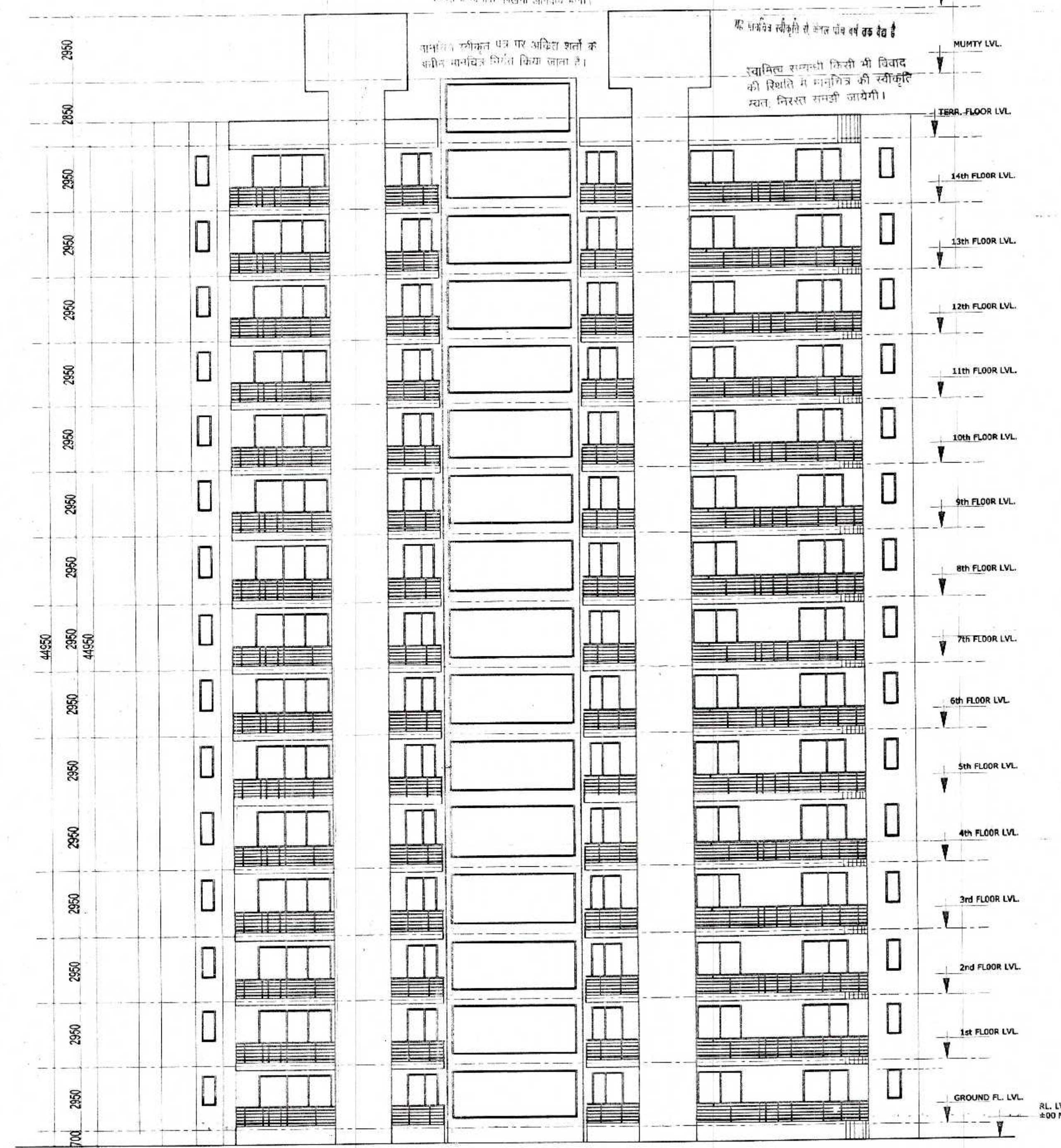
ELEVATION
